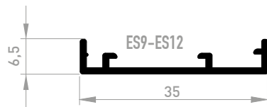
7187* COUVRE JOINT DROIT 35 mm GR. MET. Solape recto para grapa de 35 mm gr. plast.
