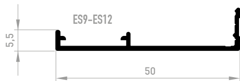
7188* COUVRE-JOINT DROIT 50 mm GR. PLAST. Solape recto 50 mm gr.plást.
