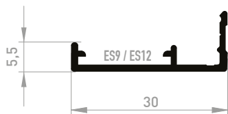
7151* COUVRE JOINT DROITE DE 30 mm Solape recto 30mm
