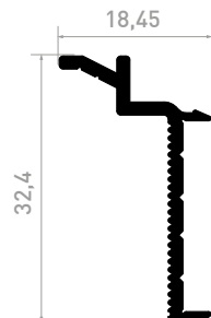
7186* PIECE D'ALUMINIUM POUR COUVRENT JOINT 7187 ET 7196 Grapa de aluminio para solapes 7187 y 7196
