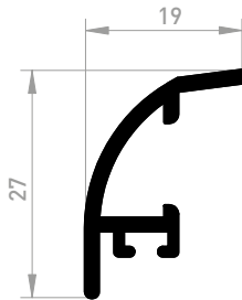
70028 REJET D'EAU CLIPPÉ Vierteaguas clipado
