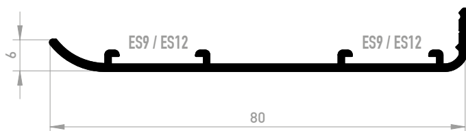
4576* COUVRE-JOINT DE 80 mm Solape de 80 mm
